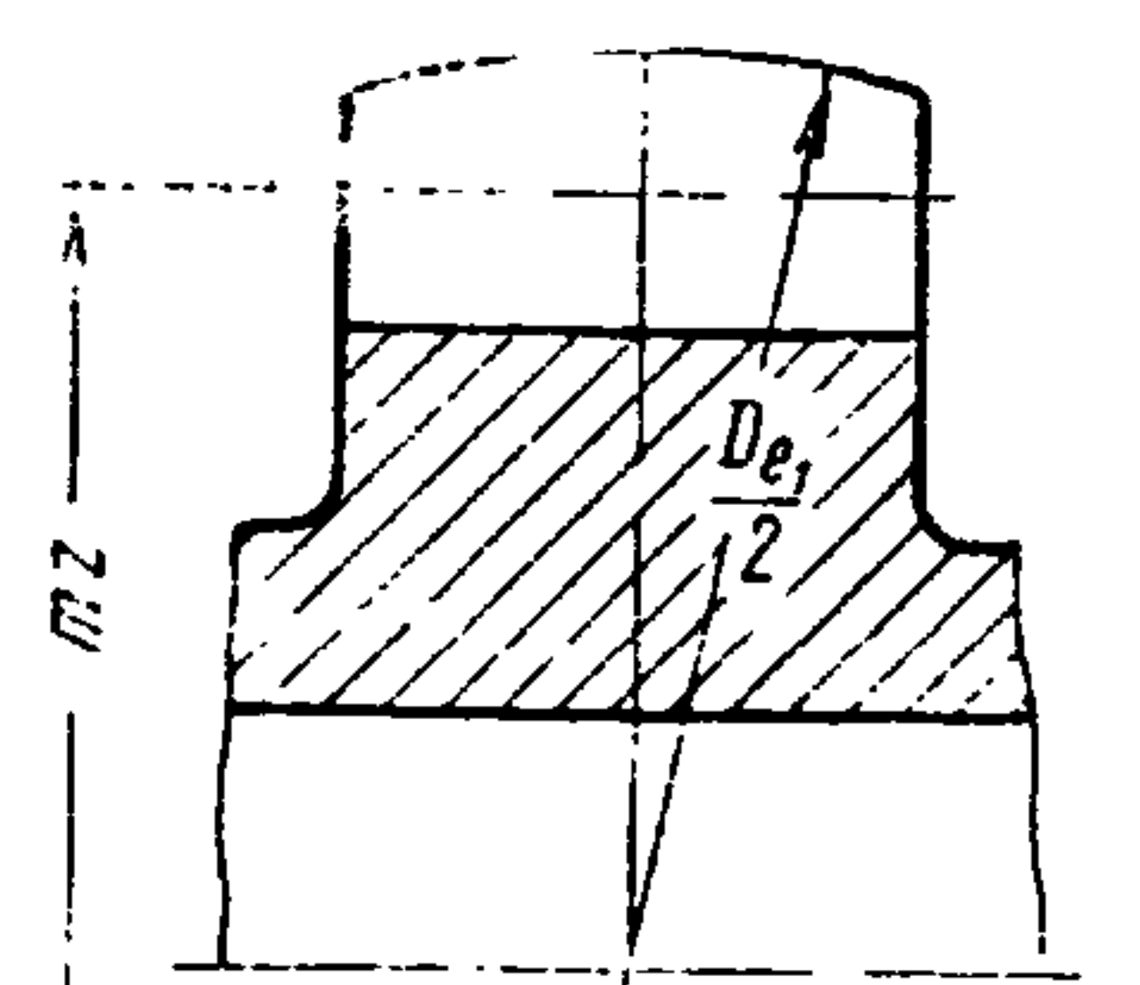
Развертка сечения зуба втулки делительным цилиндром
