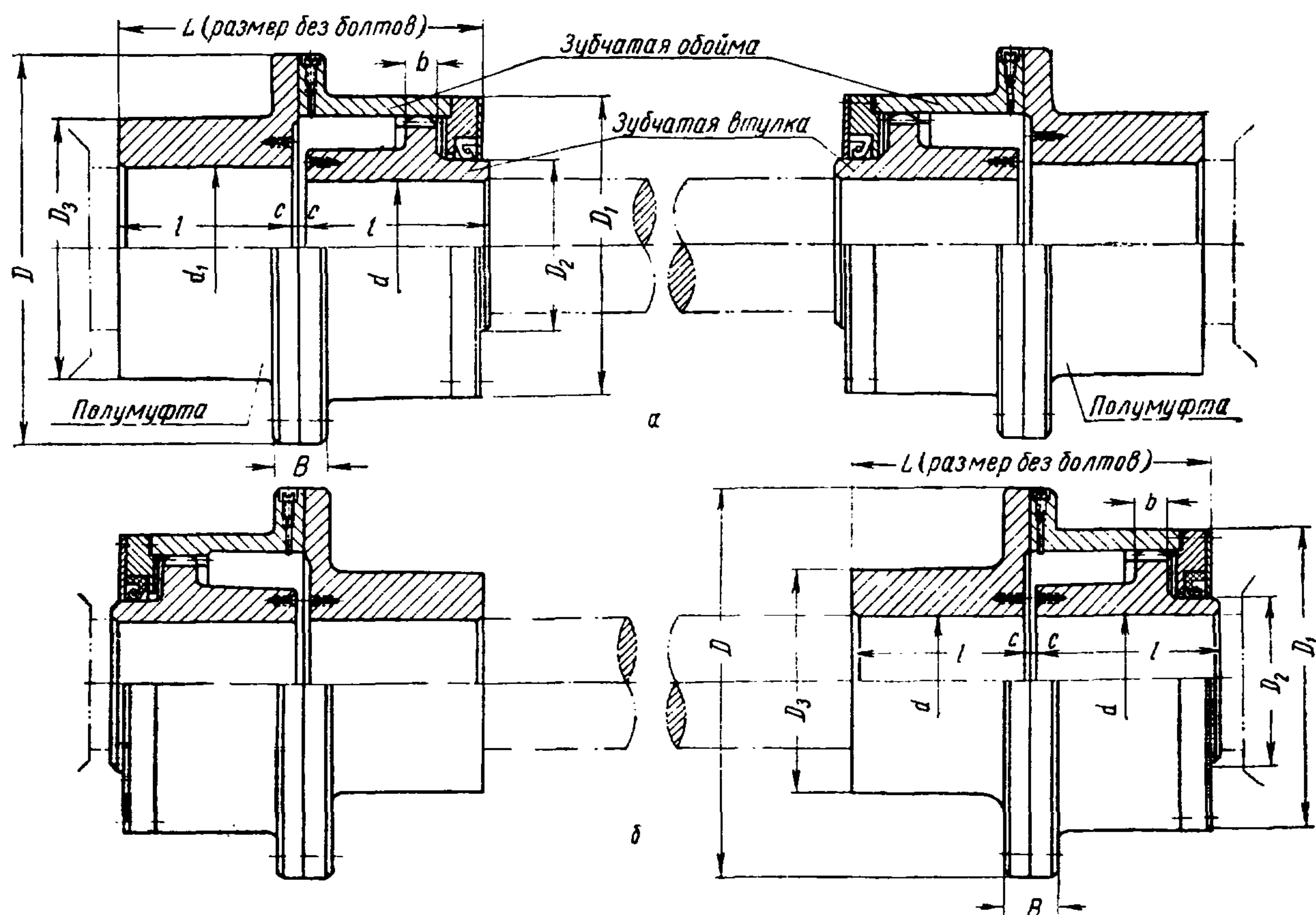
Черт. 2. Муфта типа МЗП
