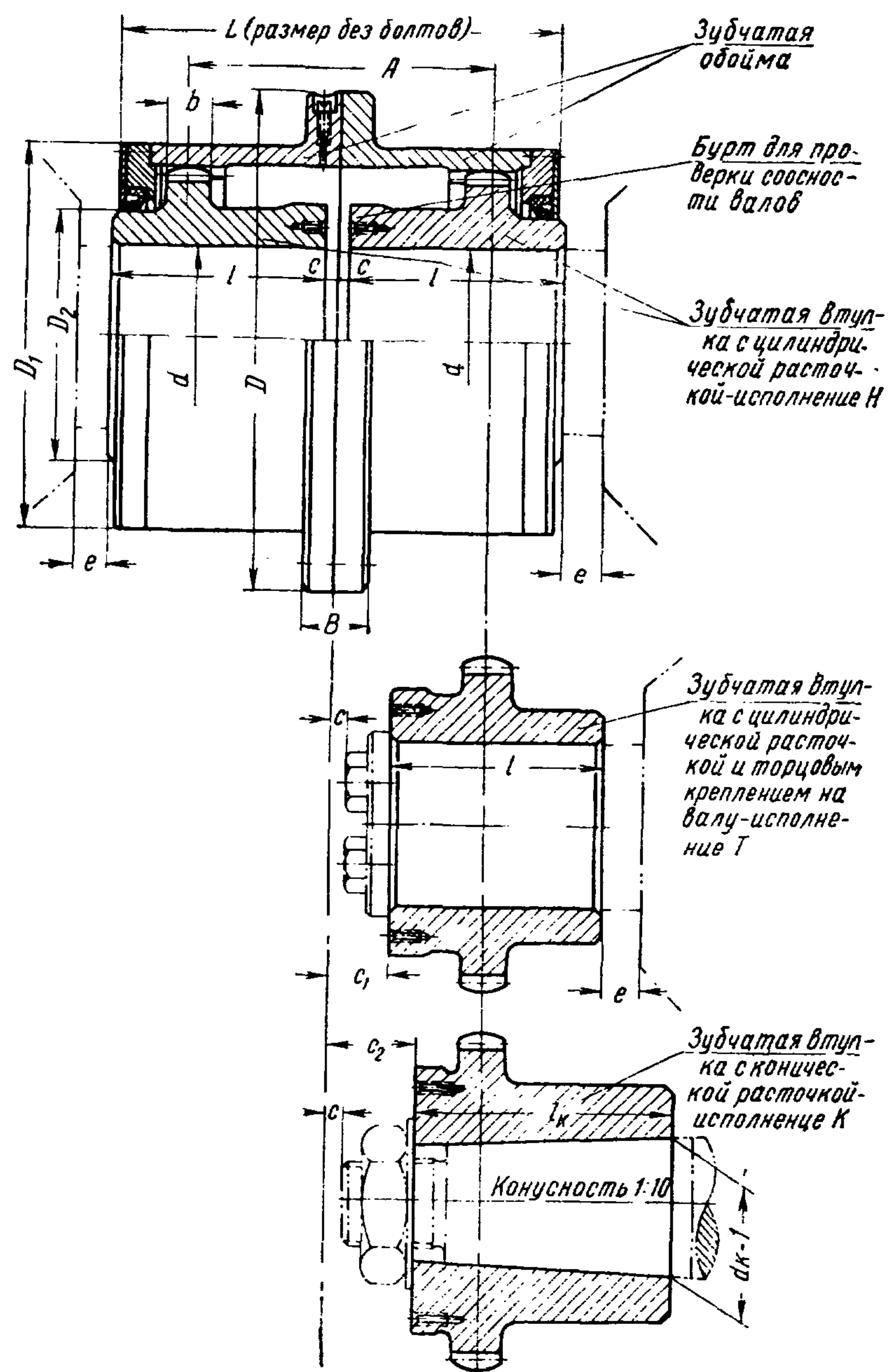
Черт. 1. Муфта типа МЗ.
