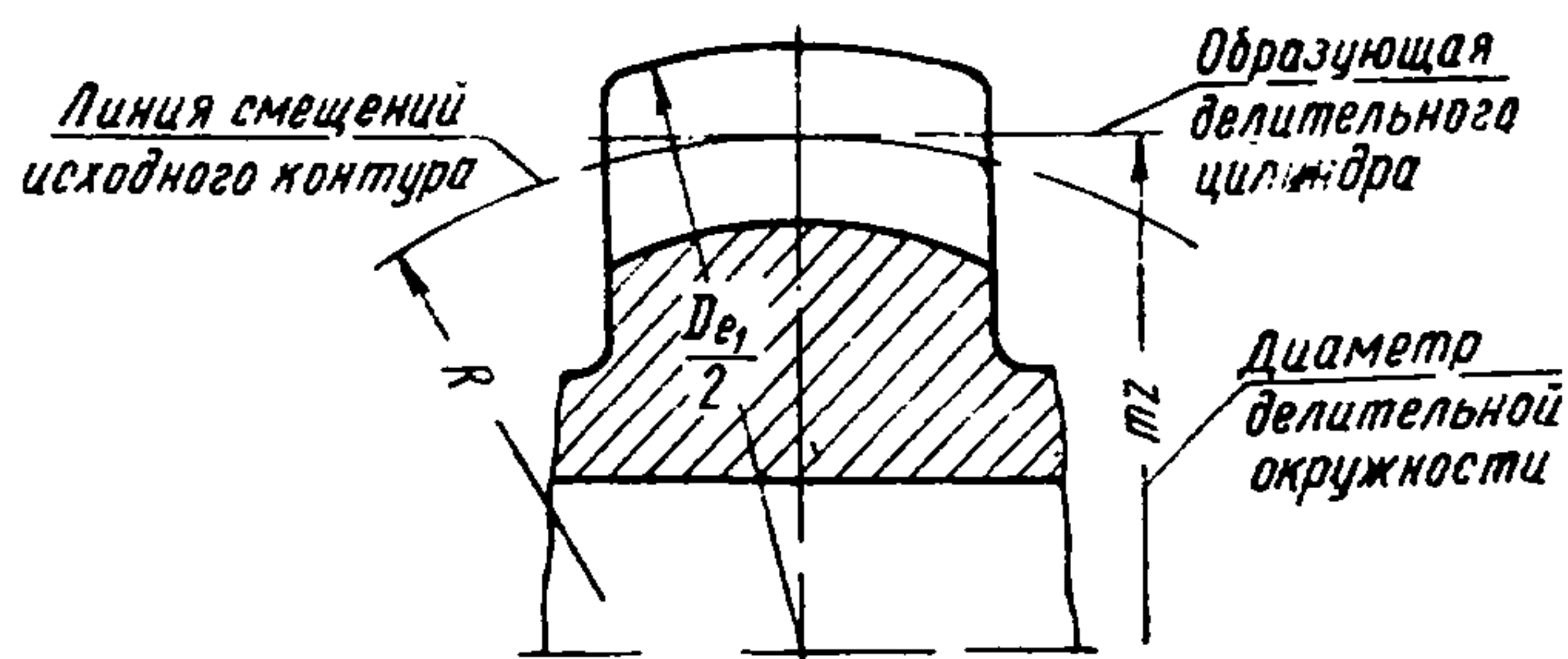
Развертка сечения зуба втулки делительным цилиндром
